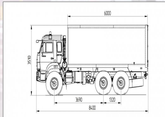
Kraftfahrzeug für Sprengmittelverkehr
