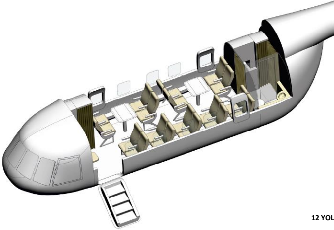
18 YOLCU KAPASİTELİ Mİ-8MTB-1 CABRİO SALON
